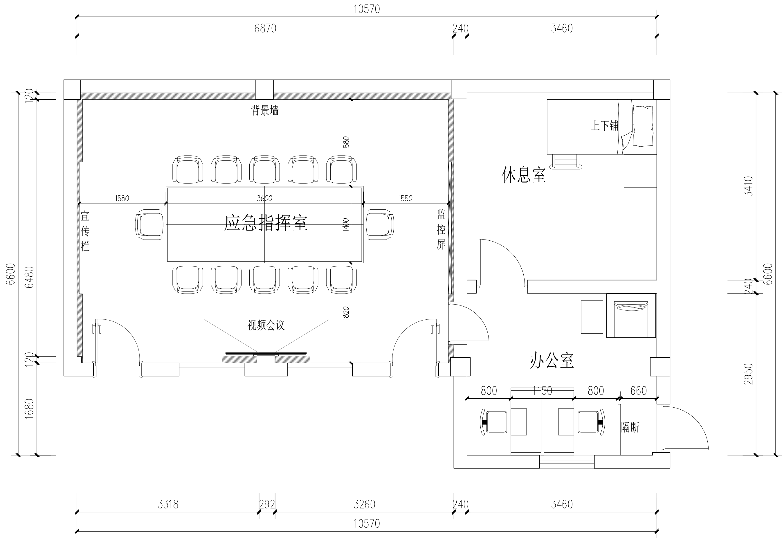
FF 赤石镇应急指挥中心平面图 比例 1:50 (A3)
