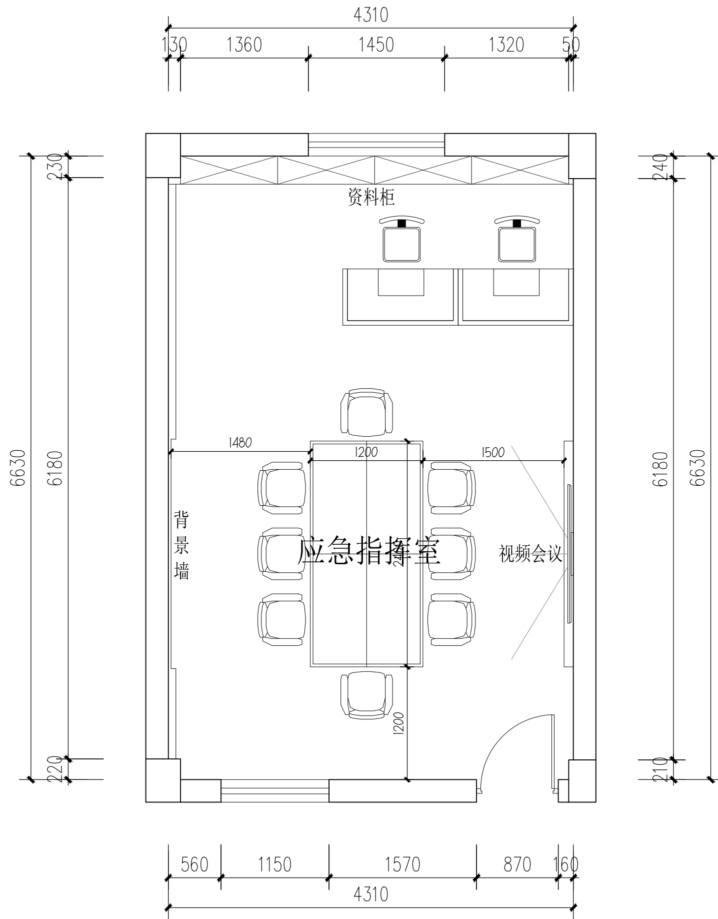
FF 鲕门镇应急指挥中心平面图 比例 1 : 50 (A3)
